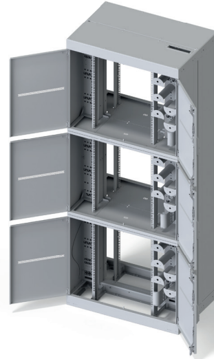
CARMA Kollokationsrack 1/3
